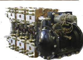
Котушки контак- торів, електропнев- матичні перемикачі
